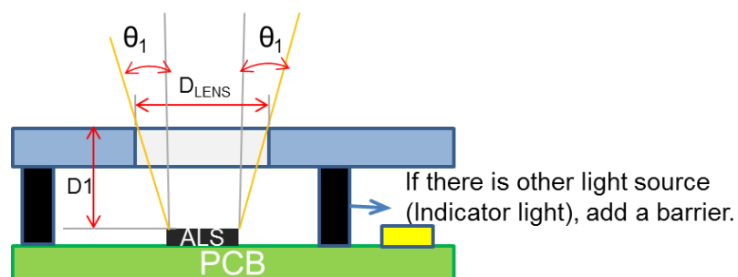
图一、朝上开孔建议
