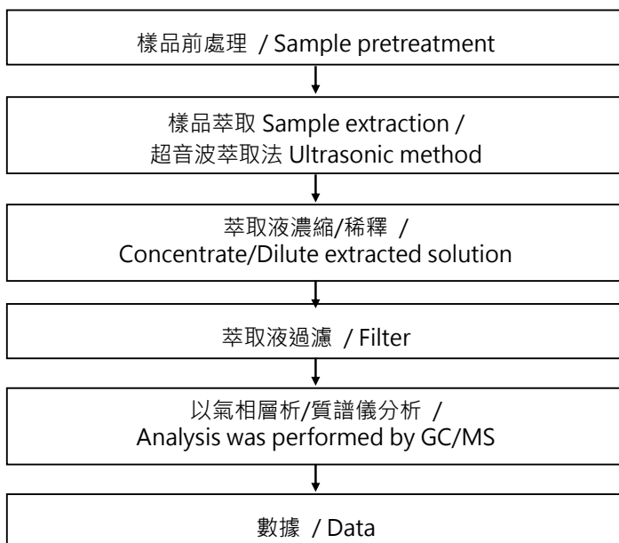
六溴環十二烷分析流程圖 / Analytical flow chart - HBCDD
